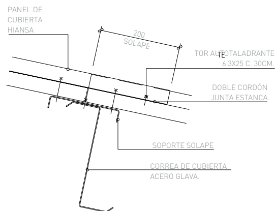
SECCIÓN SOLAPE
